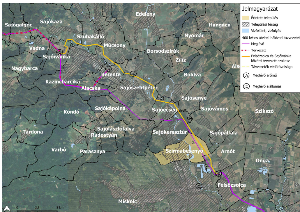
A 400 kV-os vezeték és Szirmabesenyő elhelyezkedése a tervezési területen (alaptérkép: Google Térkép)
